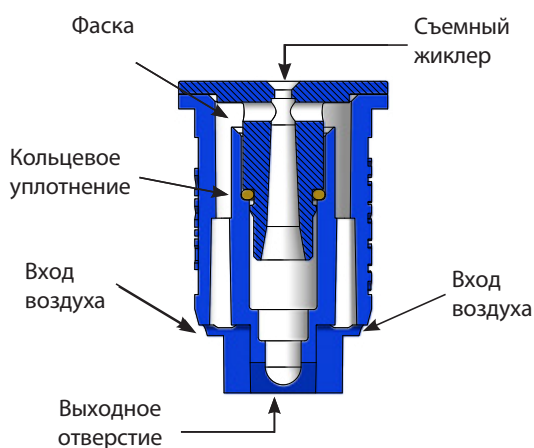
Распылительный наконечник AIXR110 VP (вид в разрезе)
